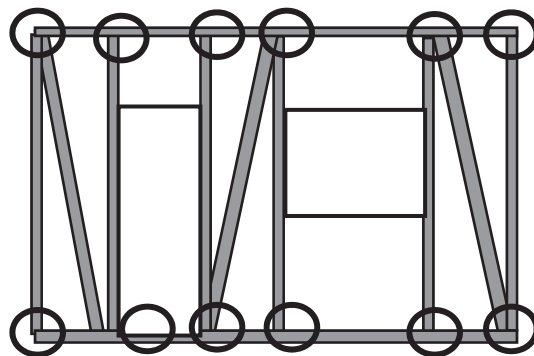
補強金物を設置
