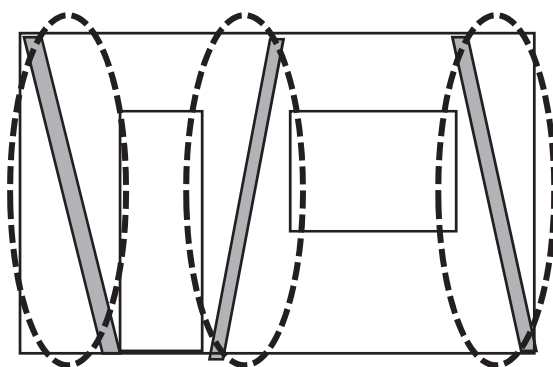
筋かいや面材で補強
